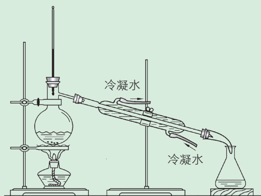
图3-4-3 蒸馏实验装置示意图
