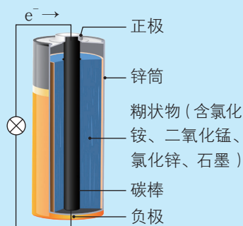
图2-2-15 酸性锌锰干电池组成示意图
