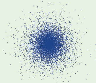
图1-1-7 氢原子的“电子云模型”
