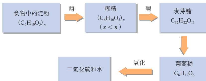
图3-3-8 淀粉在人体中的变化
