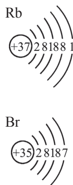
图1-2-4 铷和溴的原子结构示意图
