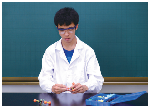
图3-1-6 学生在搭建有机化合物分子的球棍模型
