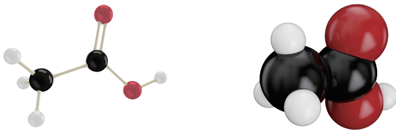
图3-3-5 乙酸分子的球棍模型和空间填充模型
