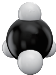
图3-1-4 甲烷分子的空间填充模型
