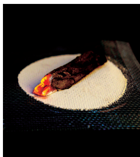
图2-2-3 木炭在空气中燃烧
