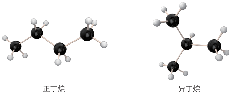
图 3-1-14 分子式为 \text{C}_4\text{H}_{10} 的烷烃的两种同分异构体的球棍模型
