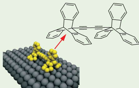
图3-1-11 分子轮
