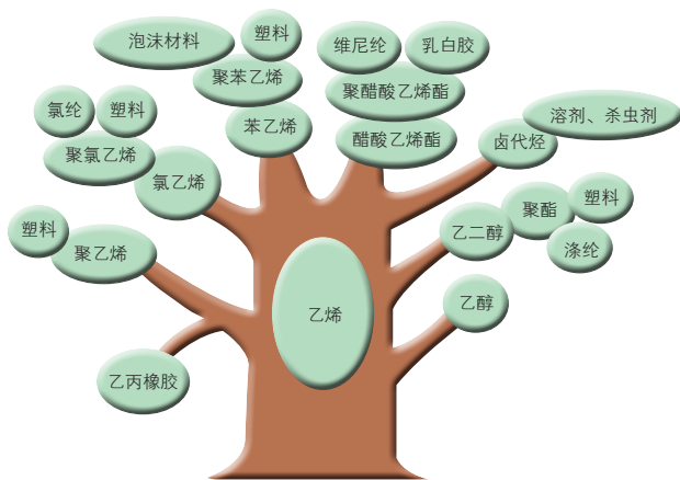
图3-2-9 乙烯用途示意图
