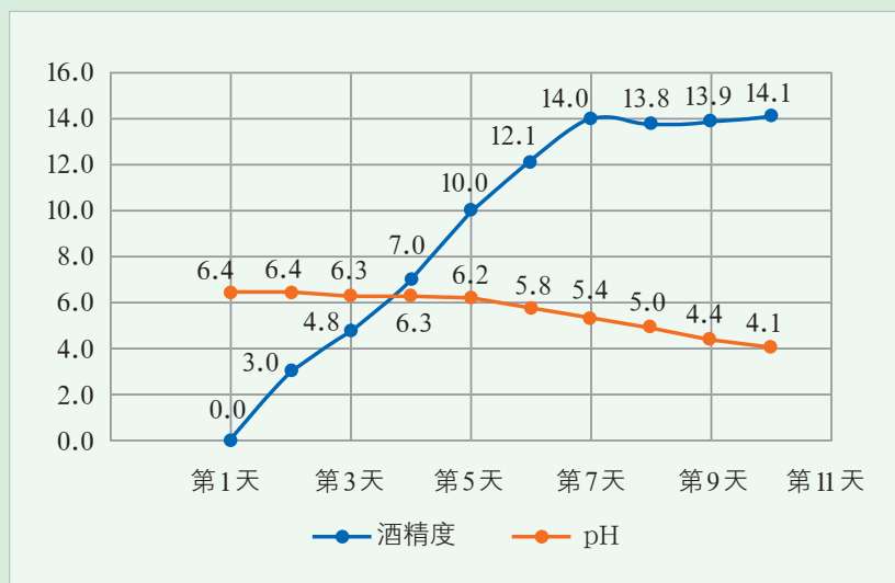
图3-4-2 自制米酒的实验数据
