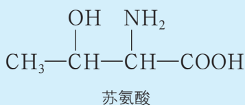
图3-3-11 人体中的几种必需氨基酸
