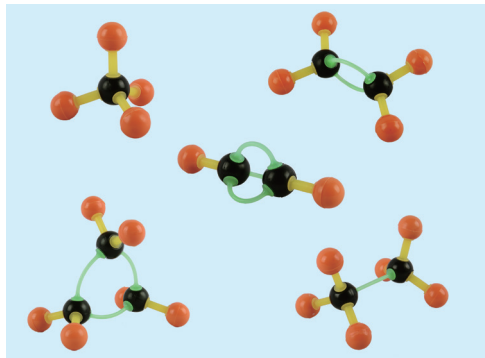
图3-1-7 学生搭建的球棍模型作品示例
